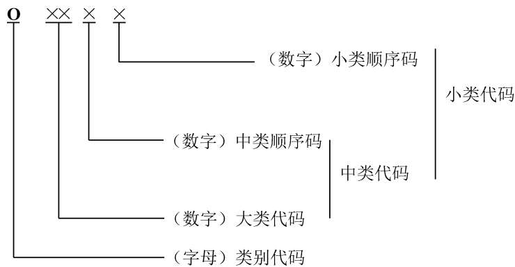
图 2 代码结构
